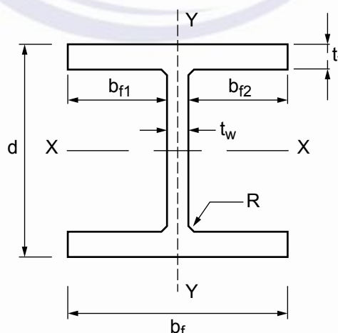
Figura F.1 – Perfil metálico
